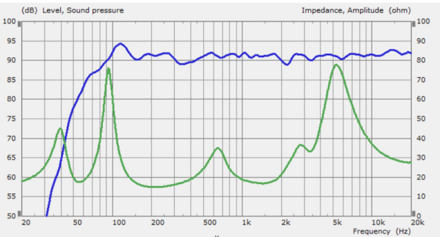
阻抗/频率响应:
