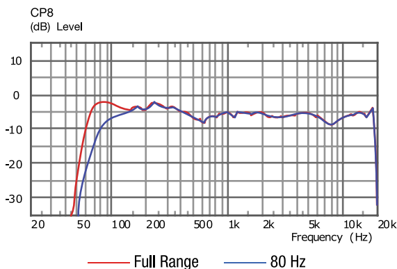
CP8 轴向频率响应
